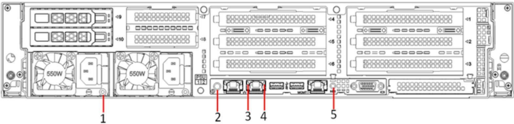
图 2-10 AR2325-TD 后面板指示灯和按钮
