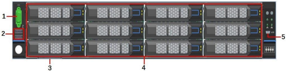
图 2-1 AR2325-TD 3.5 英寸 12盘位硬盘驱动器正面视图
