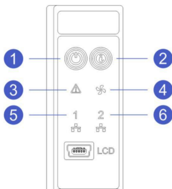
图 2-7 右控制面板连接器
