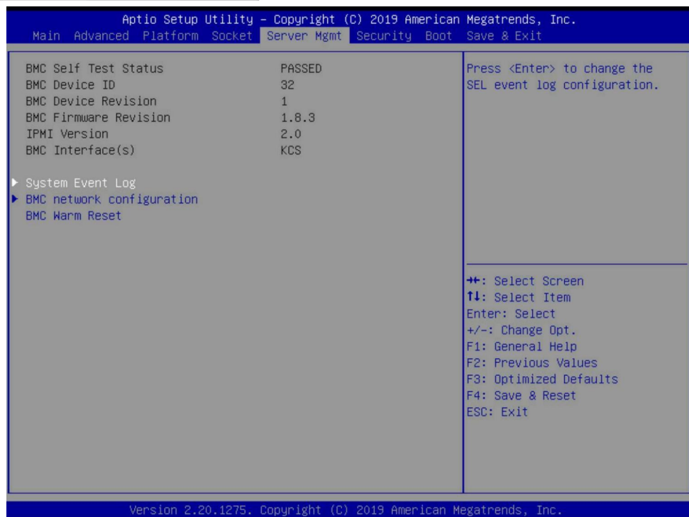
图 5-4 Server Mgmt 界面
