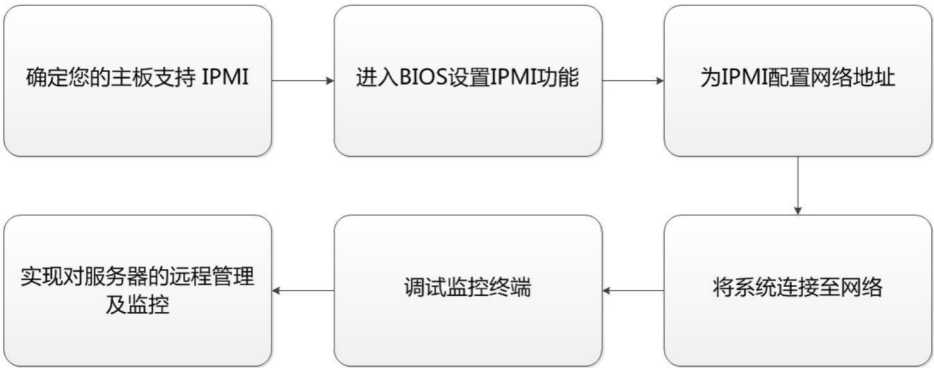
图 5-1 IPMI 部署流程
