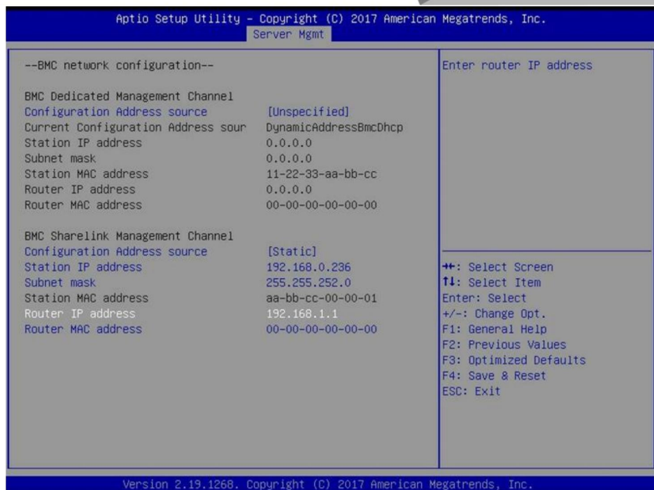
图 5-7 Static 模式设置
