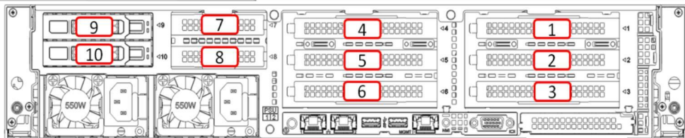
图 2-9 AR232-TD PCIe 插槽分布后视图
