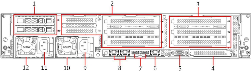
图 2-8 AR2325-TD 系统背面视图
